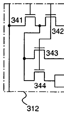
FIG. 12E
