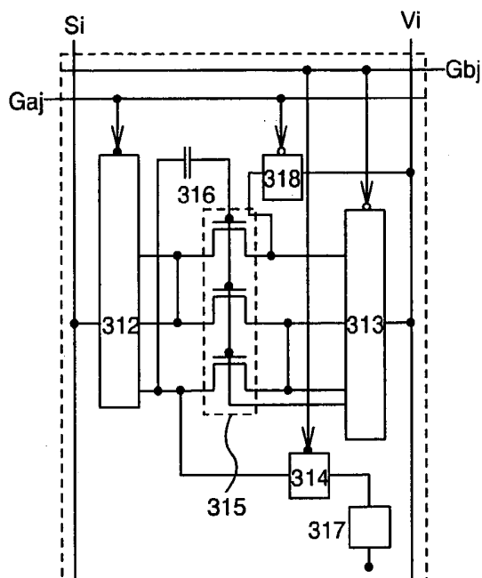
FIG. 15A
