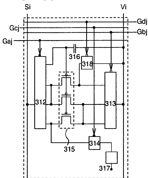
FIG. 13C
