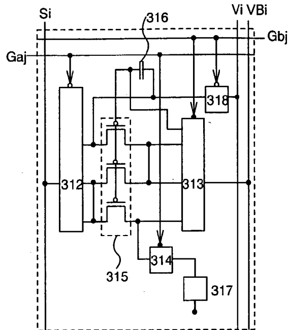
FIG. 15B
