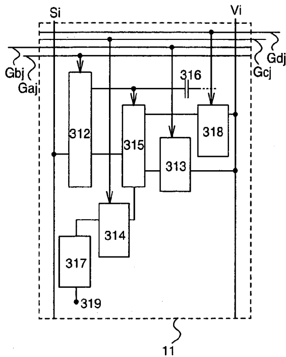
FIG. 11C
